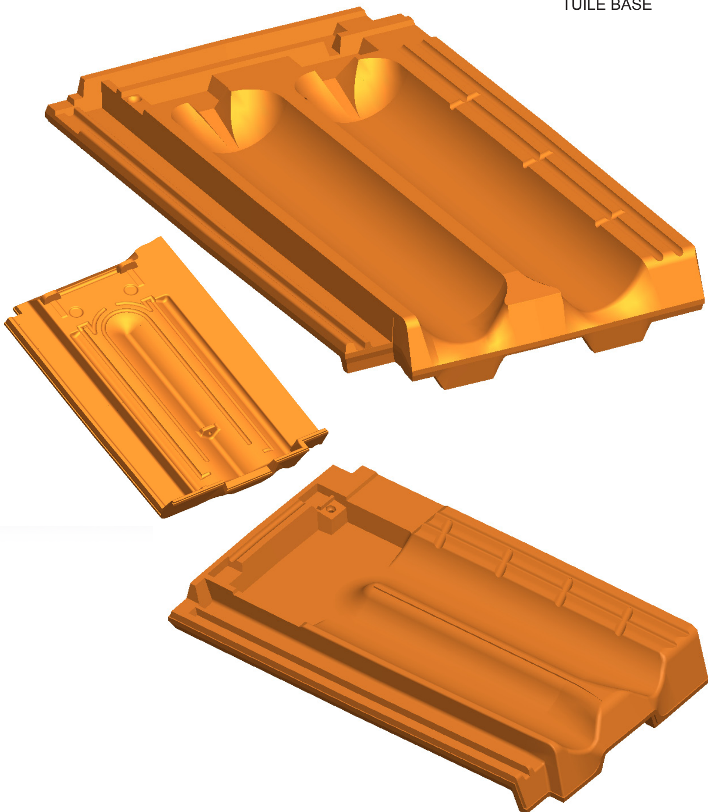
TUILE BASE
