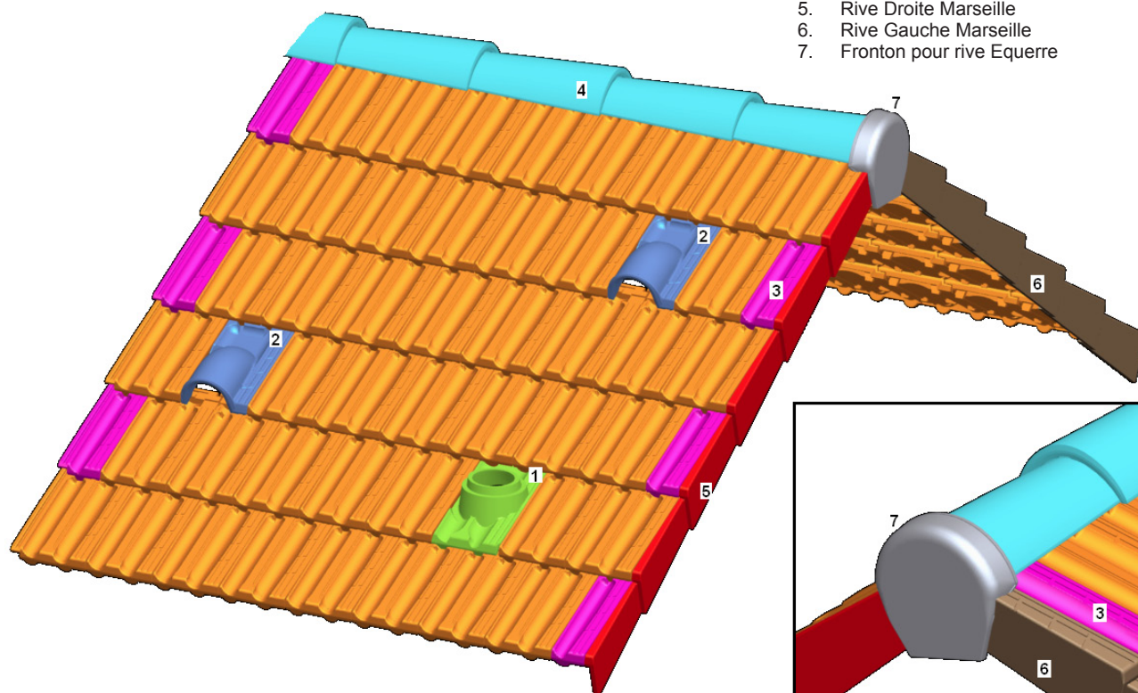
ACCESSOIRES AU TOIT
